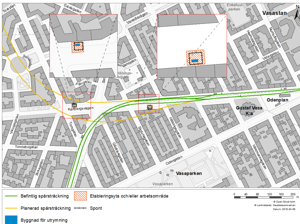
Figur 28. Byggnader för utrymning på sträckan Odenplan till Hagastaden.
