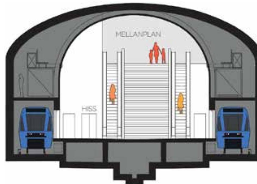
Figur 19 Typstation i tvärsnitt, framtagen av förvaltning av utbyggd tunnelbana (FUT).
