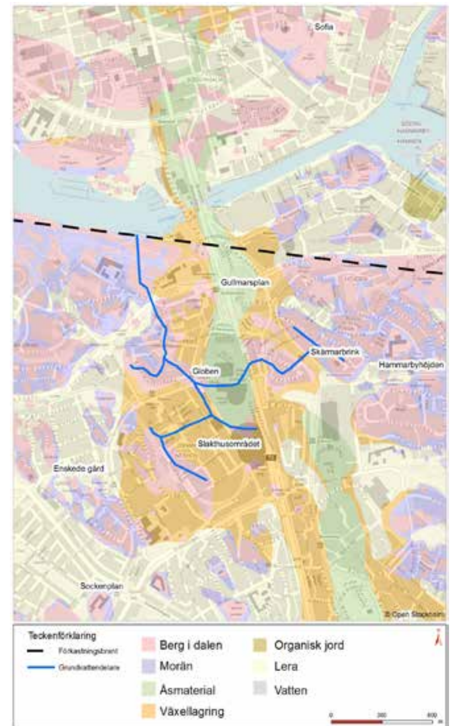
Figur 12 Karta över grundvatten och jordarter. Enkel blå linje visar grundvattendelare, svart streckad linje visar förkastningsbrant. (SGU jordartskarta, 2015)
