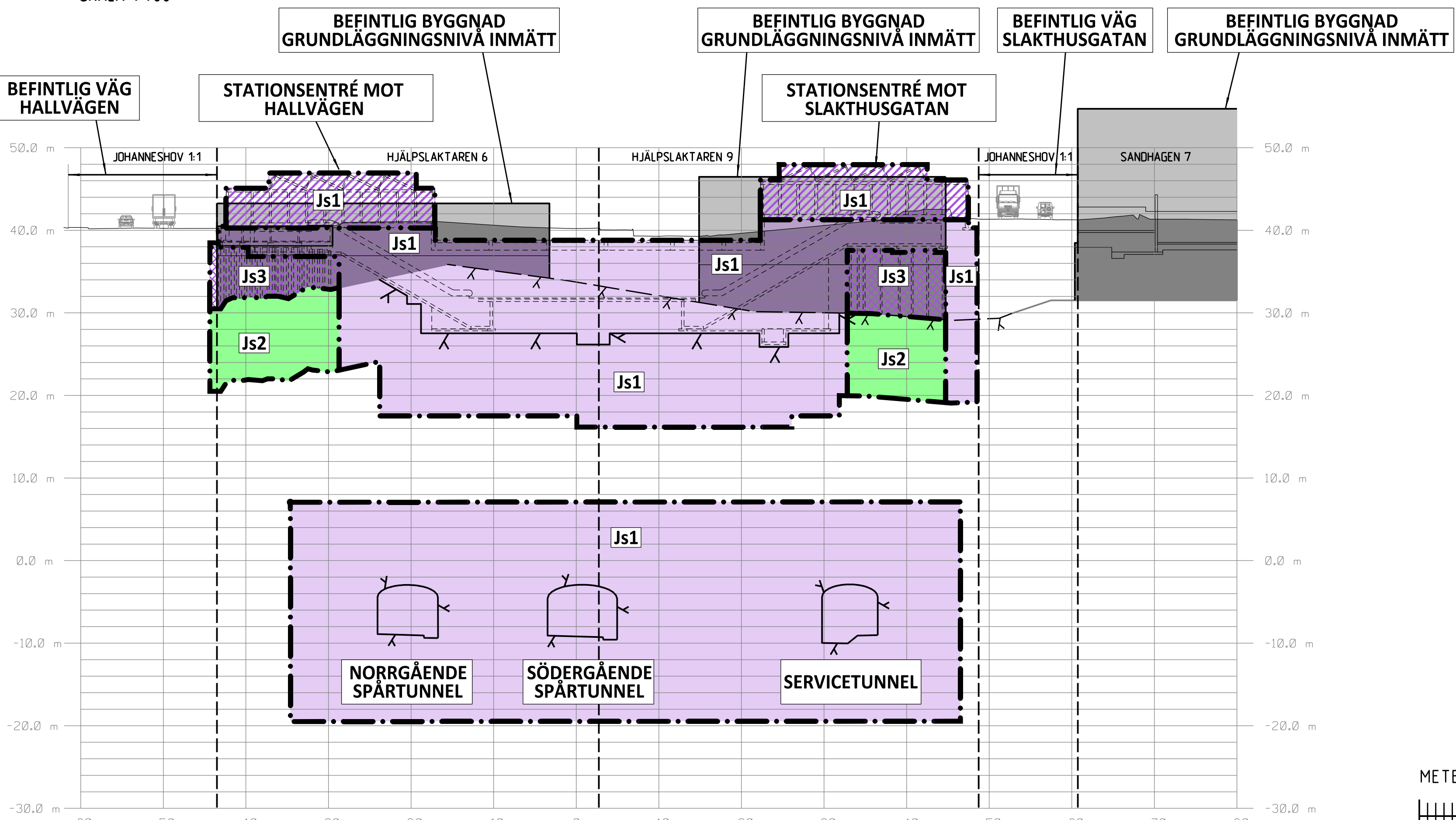
SEKTION S 4+475 SKALA 1:400
