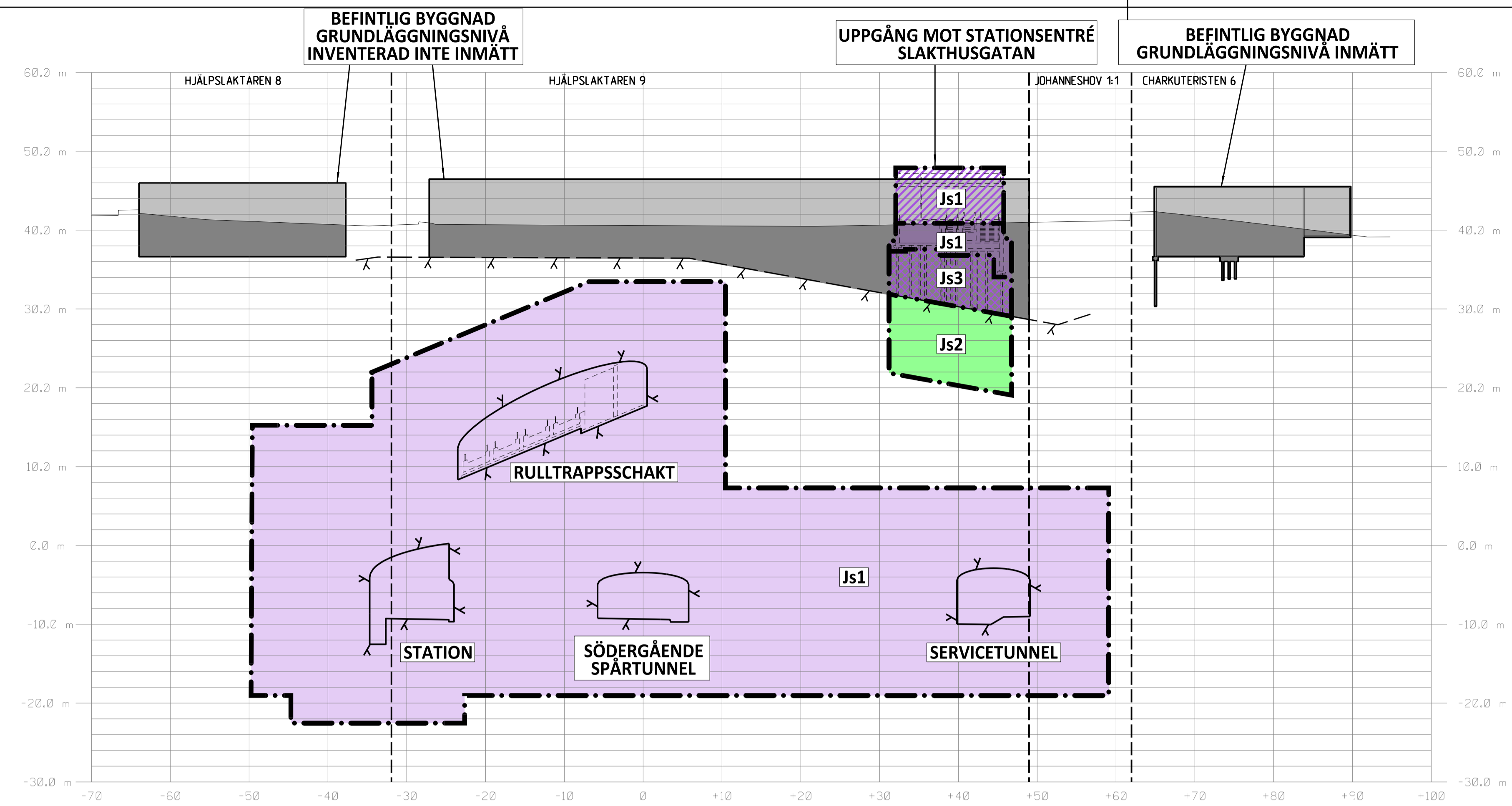
SEKTION S 4+757 SKALA 1:400
