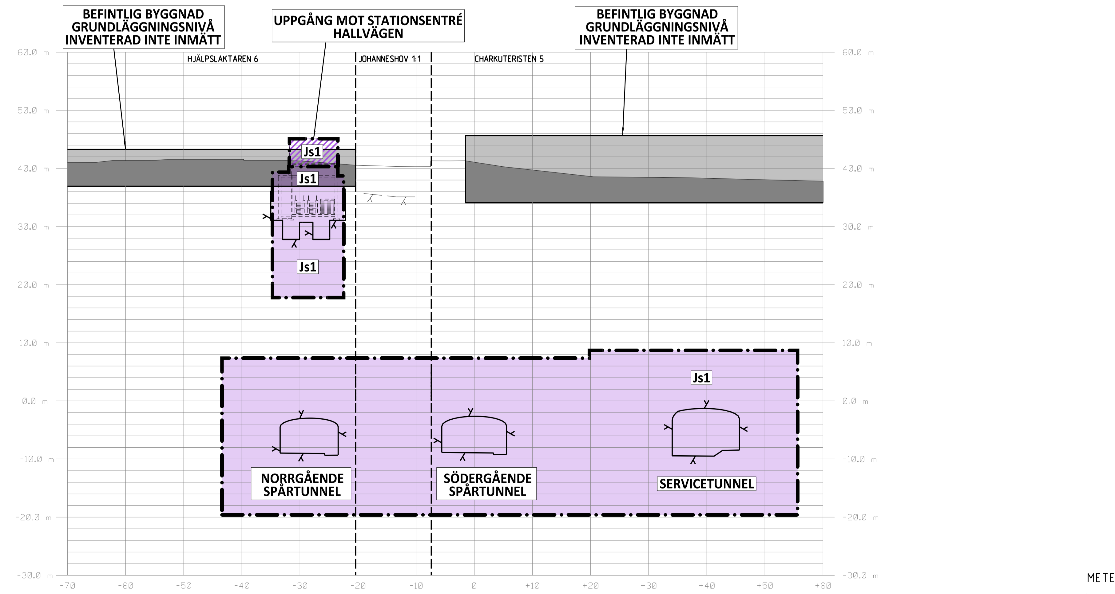
SEKTION S 4+843 SKALA 1:400
