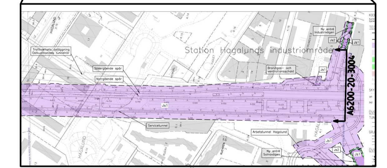
REDDVISAD TVÄRSEKTION I PLAN
