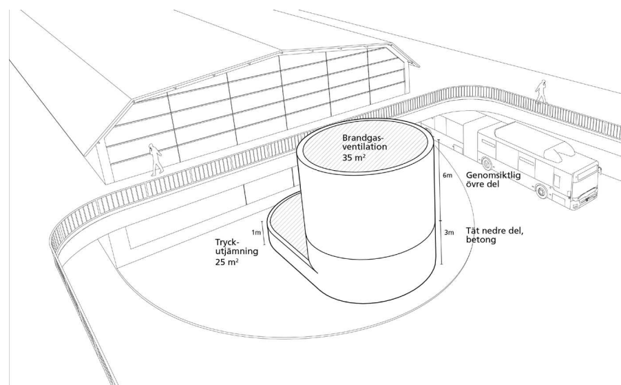
Figur 4.25 Illustration över ventilationstorn i Akalla.
