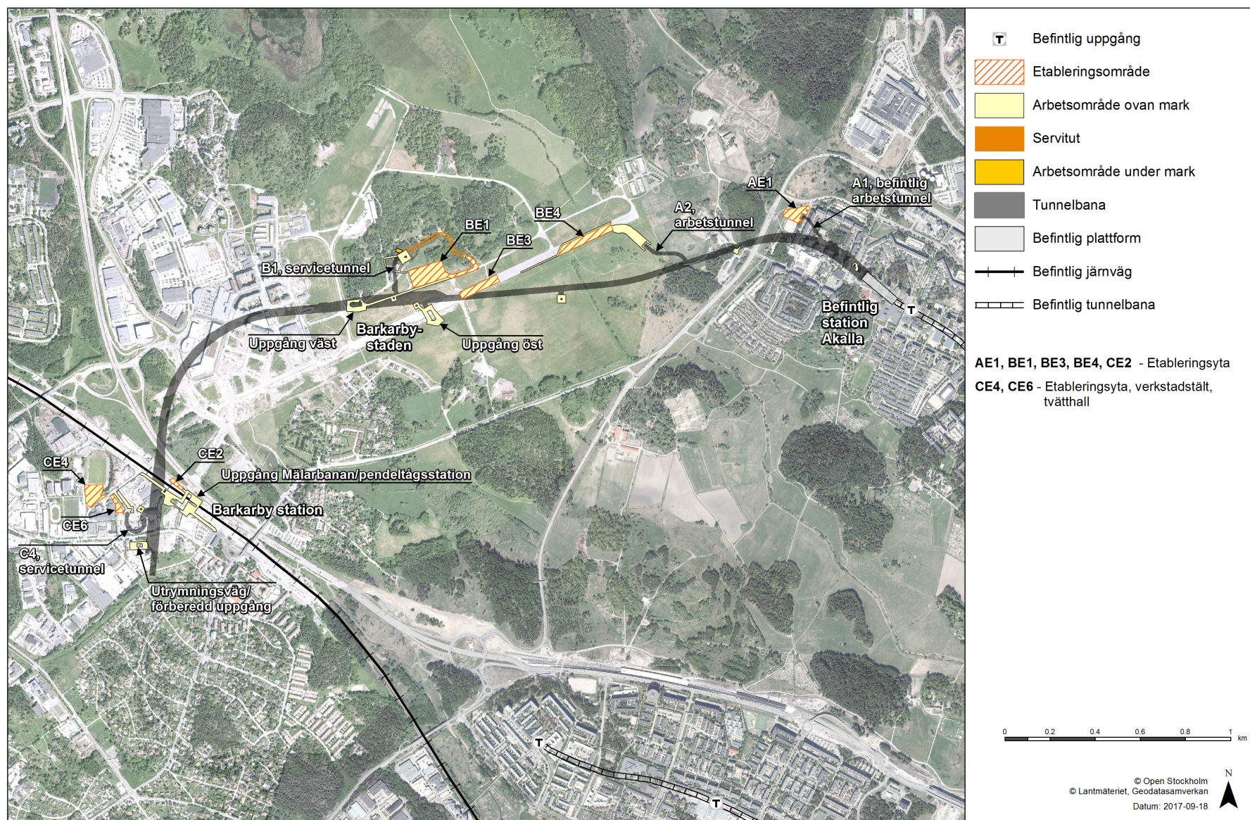
Figur 4.24 Ytor som behövs under byggskedet.
