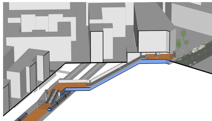
Figur 4.12 Illustration över rulltrappor och hissar uppgång öst.
