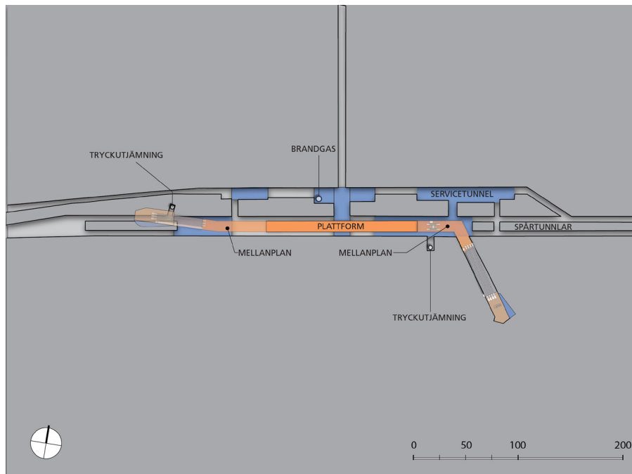
Figur 4.9 Rumslig illustration av station Barkarbystaden.
