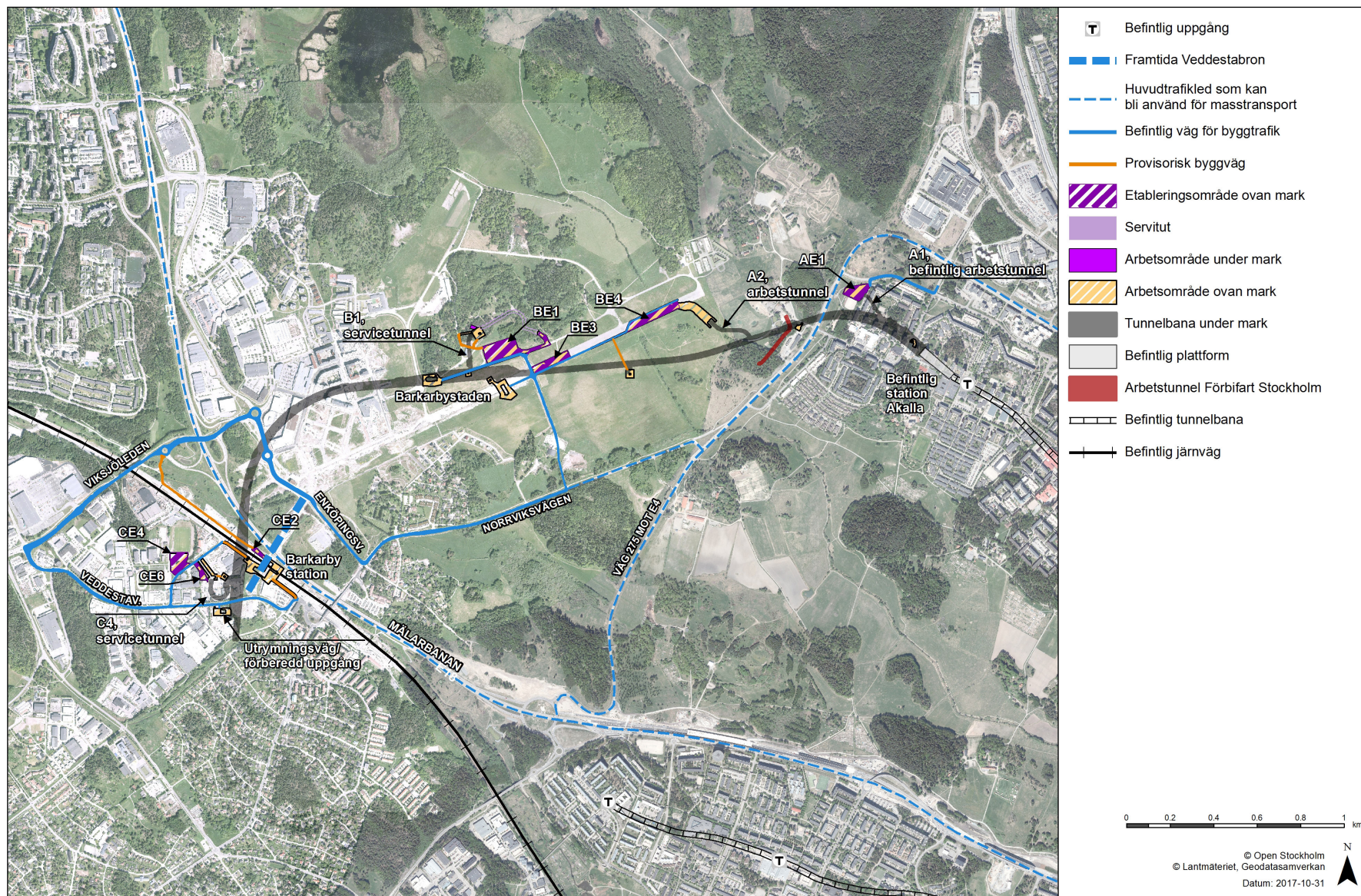
Figur 4.23 Arbets- och servicetunnlar. Genom samordning har det setts till att områdena inte ligger på samma ytor som Förbifart Stockholm.
