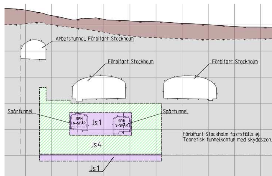
Figur 7.3 Illustrationsritning i sektion som redovisar att inom delar av skyddszon för Förfart Stockholm gäller även planbestämmelse Js4.
