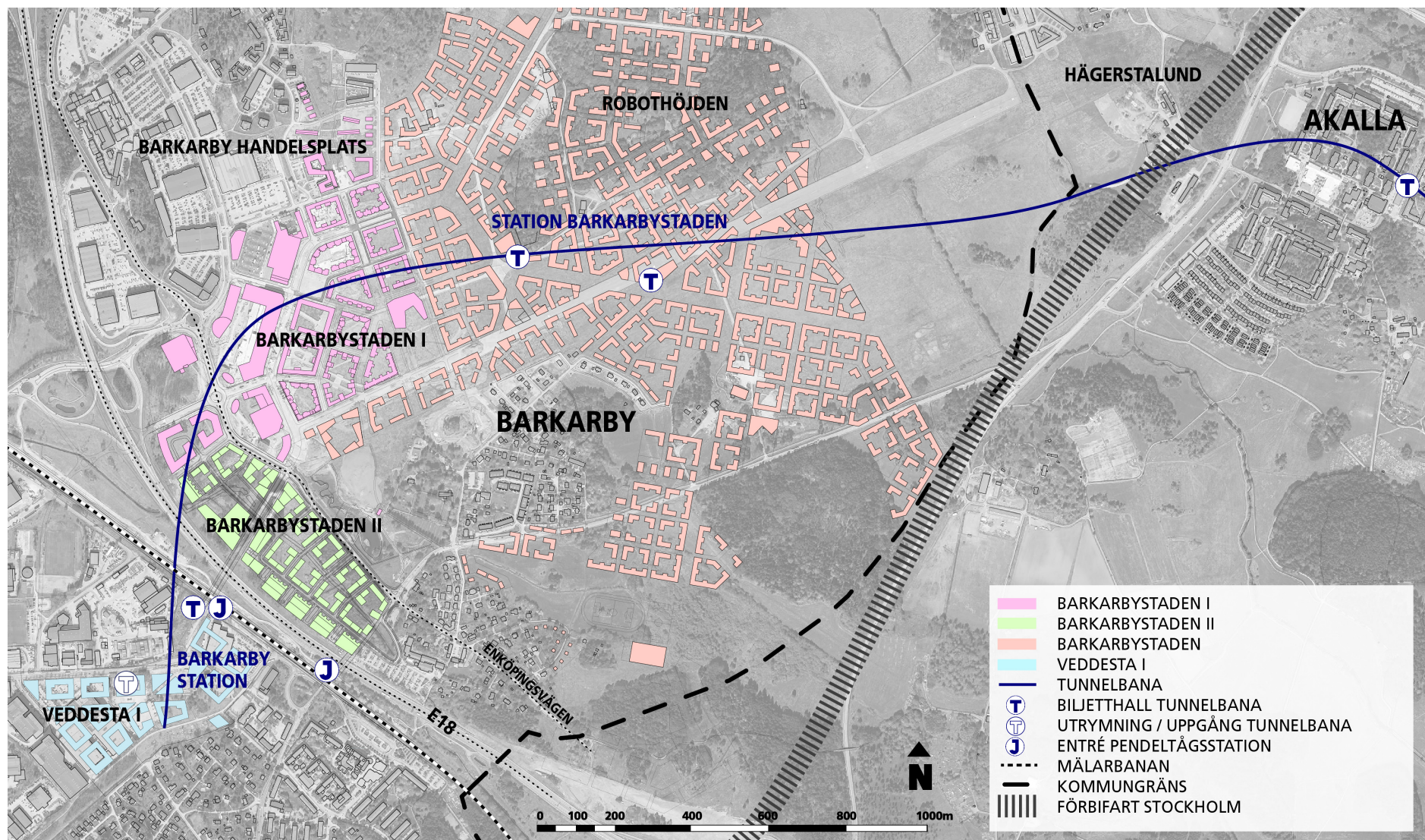
Figur 1.2 Planerad tunnelbanesträckning och stationslokalisering. Stadsutveckling pågår i Barkarby staden vilket föranleder att strukturer förändras kontinuerligt.
